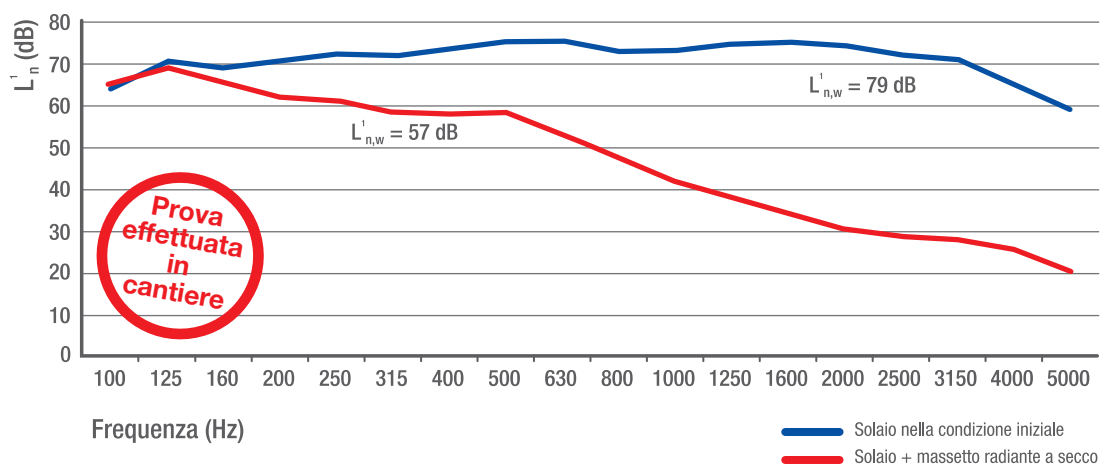
Test comparativo isolamento rumore tra locali sovrapposti con PV50
